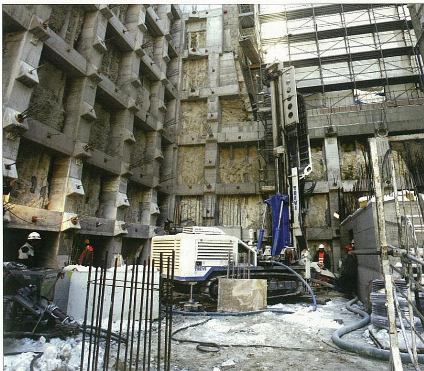
Per collocare la perforatrice sul piano di lavoro, situato a quota -9 m dal piano stradale, è stato necessario sollevare la perforatrice mediante un'autogrù da 300 t
