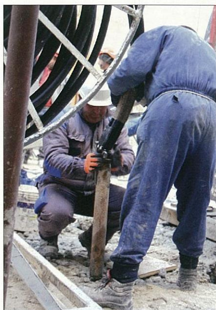
I tubi di polietilene delle sonde geotermiche vengono cementati all'interno del foro con miscele cementizie ad alta conduttività termica per favorire lo scambio col terreno
